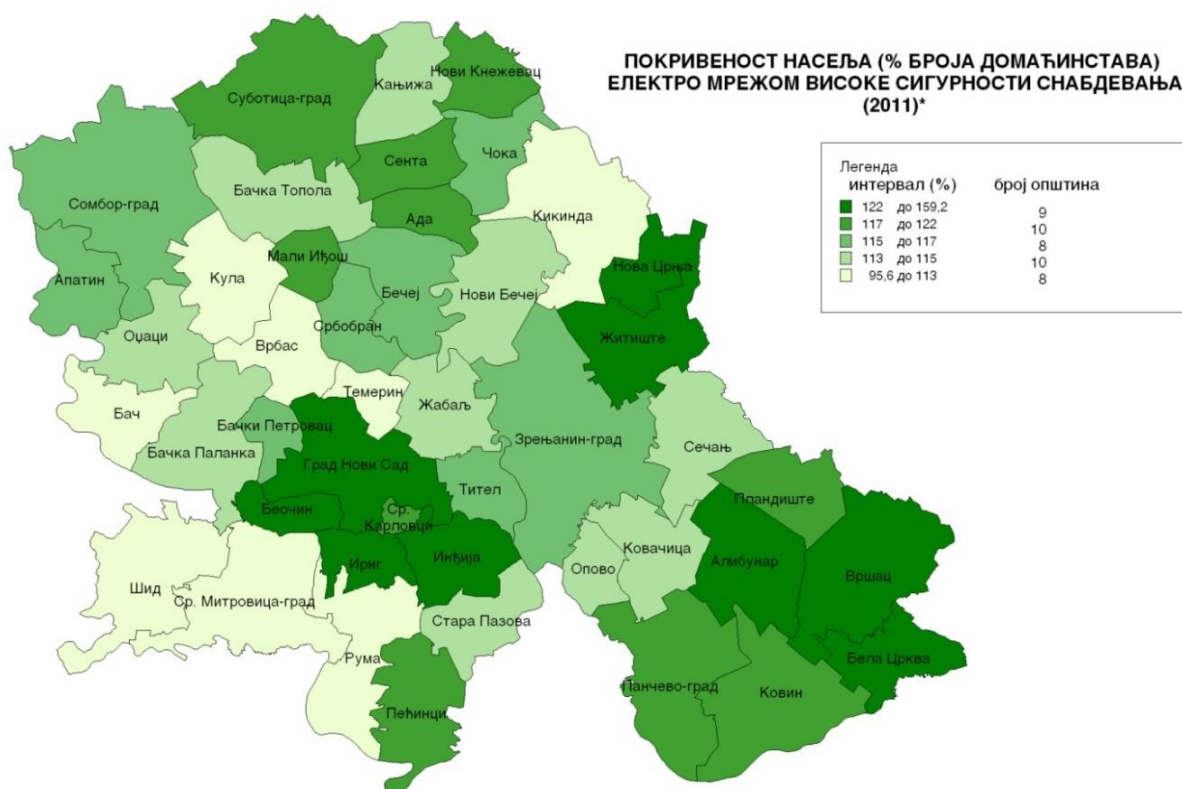
Карта 34: Покривеност насеља (% броја домаћинстава)* електроенергетском мрежом високе сигурности снабдевања - приказ по општинама/градовима
