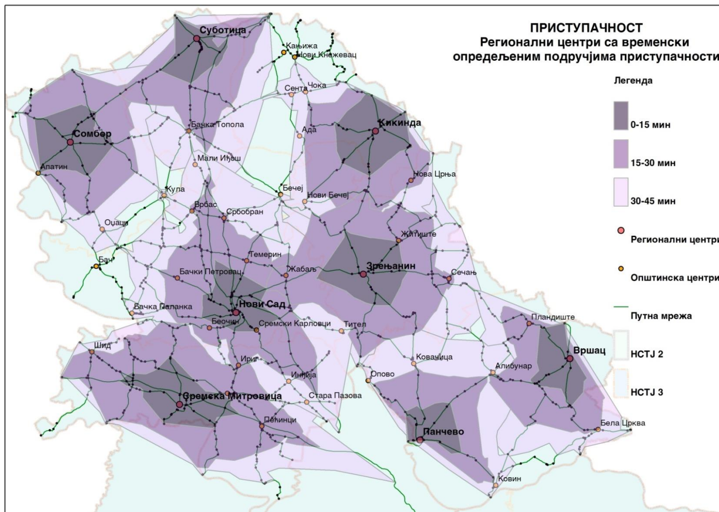
Карта 27: Регионални центри са временски опредељеним подручјима приступачности
