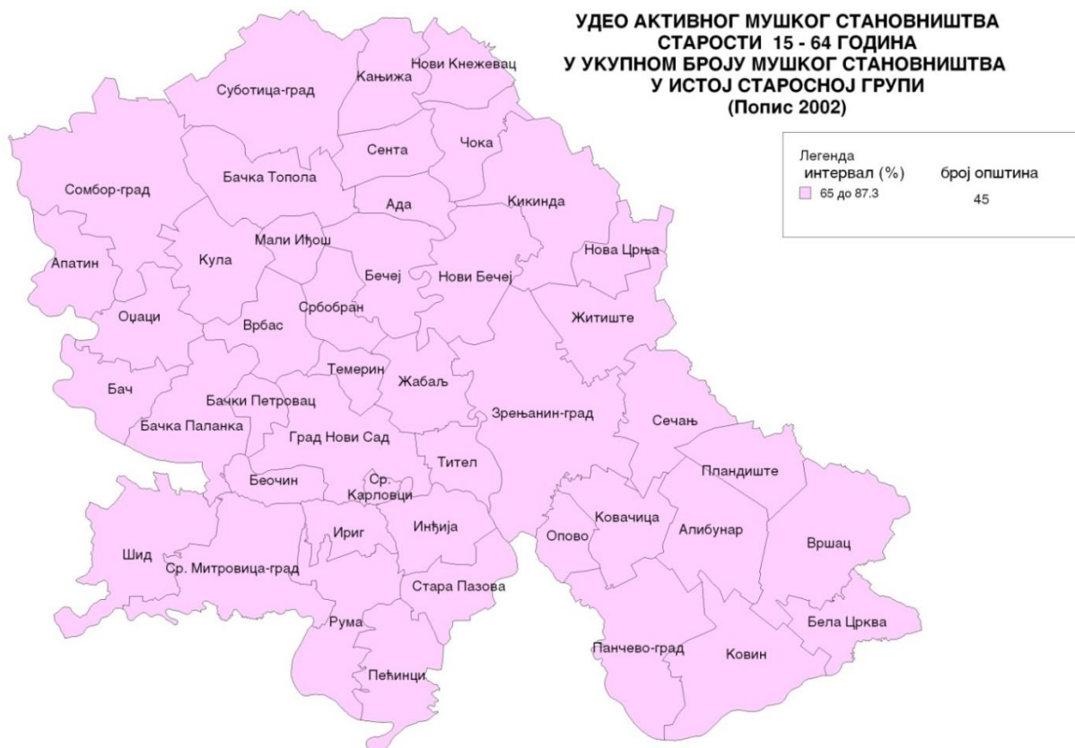
Карта 17: Стопа активности мушке популације (15-64 година) - приказ по општинама/градовима
