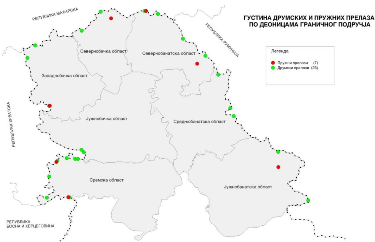
Карта 69: Густина друмских и пружних прелаза по деоницама граничног подручја (бр. прел. / 100 km) - приказ по областима
