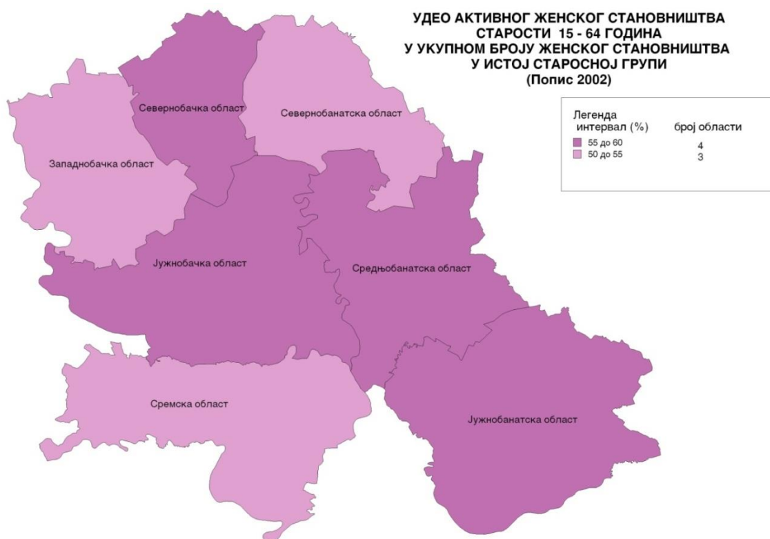
Карта 18: Стопа активности женске популације (15-64 година) - приказ по областима
