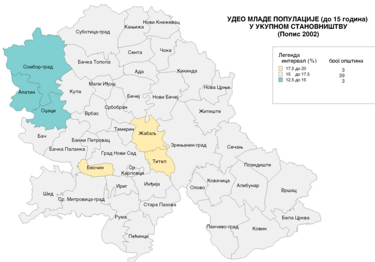
Карта 5: Удео младе популације - приказ по општинама/градовима
