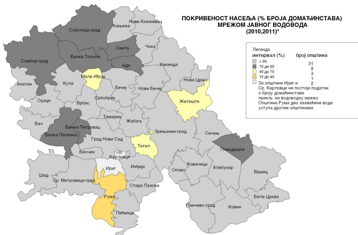
Карта 30: Покривеност насеља (% броја домаћинстава) мрежом јавног водовода - приказ по општинама/градовима
