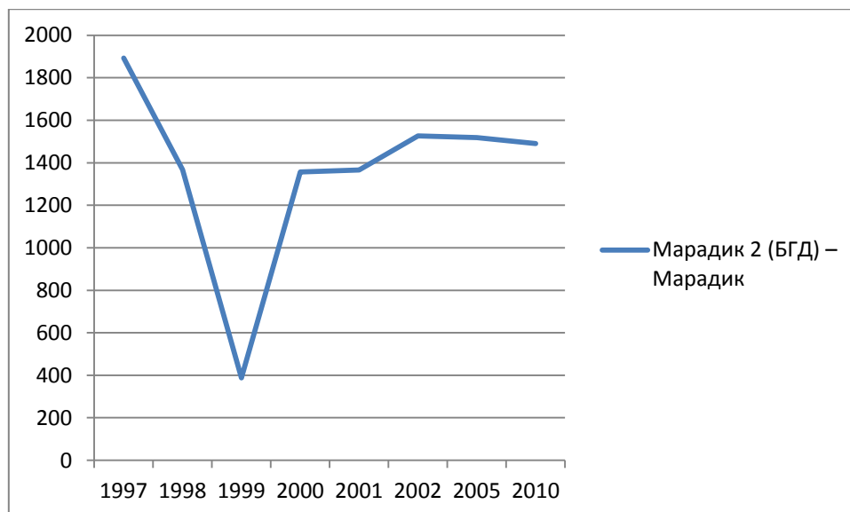
Стање саобраћајног оптерећења на државном путу I реда бр.24 по годинама (ПГДС) (воз/24h)
