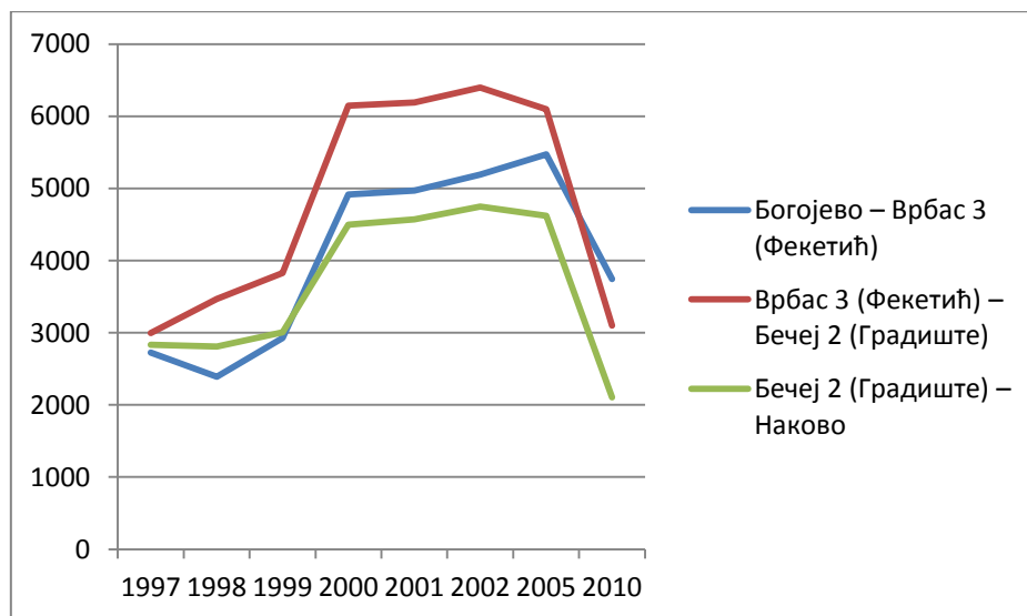
Стање саобраћајног оптерећења на државном путу I реда бр.7 по годинама (ПГДС) (воз/24h)
