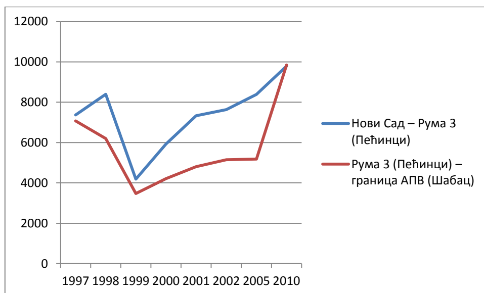
Стање саобраћајног оптерећења на државном путу I реда бр.22 ( Е-75 ) по годинама (ПГДС) (воз/24h)
