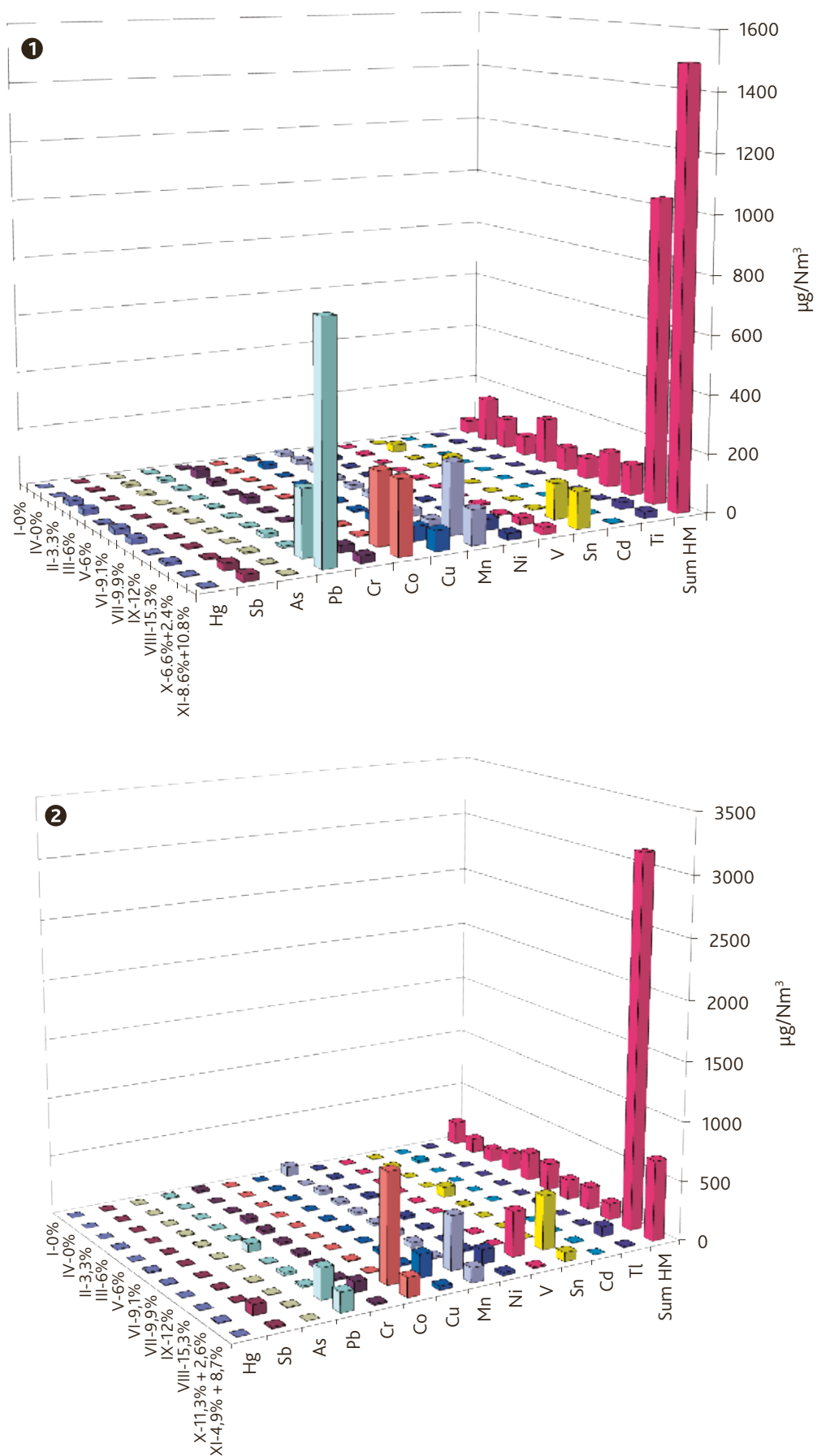
Слика 23. Емисије тешких метала на мерним местима 1 и 2 у зависности од топлотног удела отпадних гума и отпадног уља у гориву
