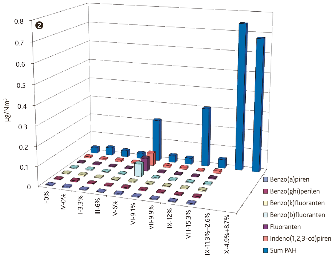
Слика 24. Емисије полицикличних ароматичних угљоводоника на мерним местима 1 и 2 у зависности од топлотног удела отпадних гума и отпадног уља у гориву
