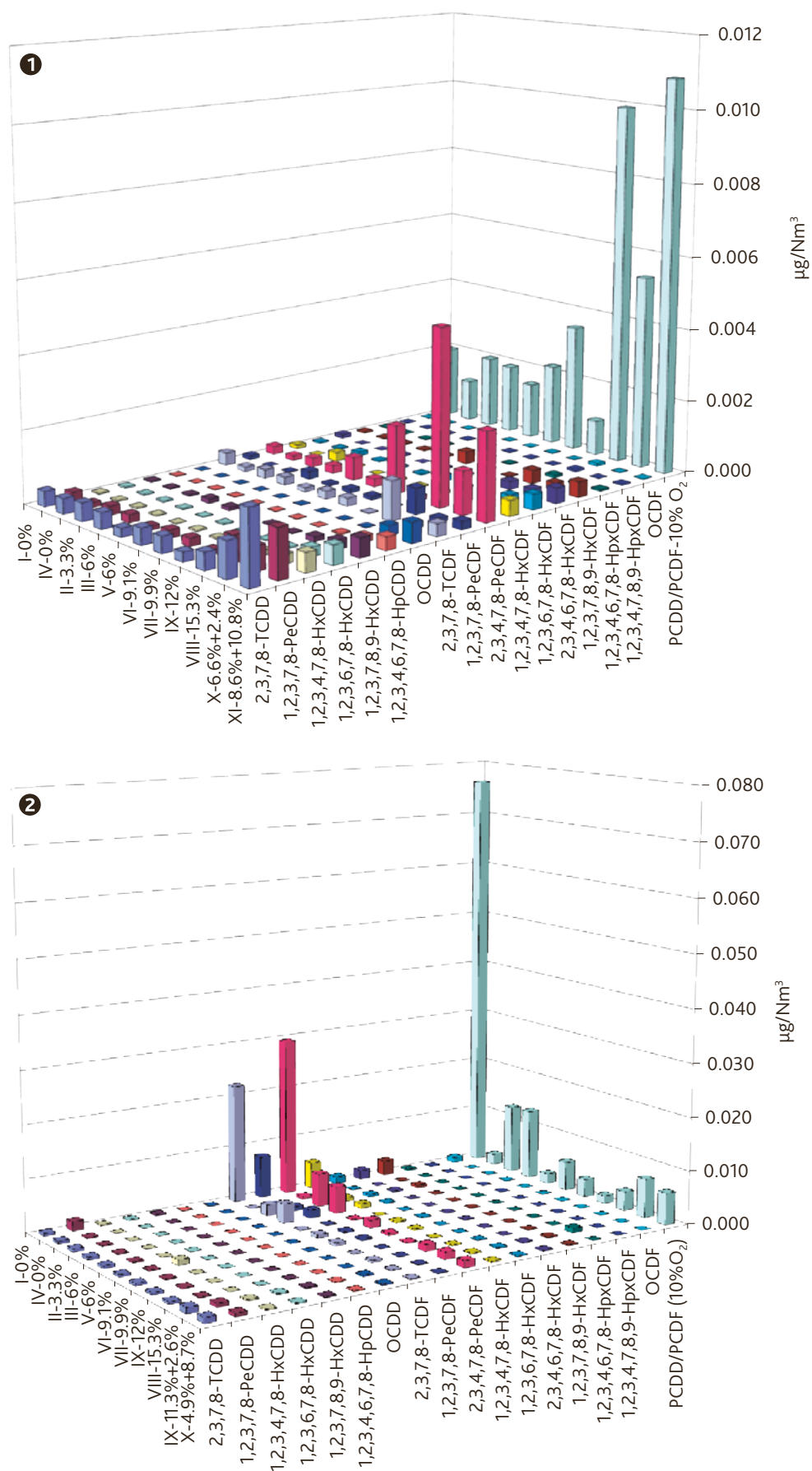
Слика 25. Емисије диоксида и фурана PCDD/PCDF на мерним местима 1 и 2 у зависности од топлотног удела отпадних гума и отпадног уља у гориву
