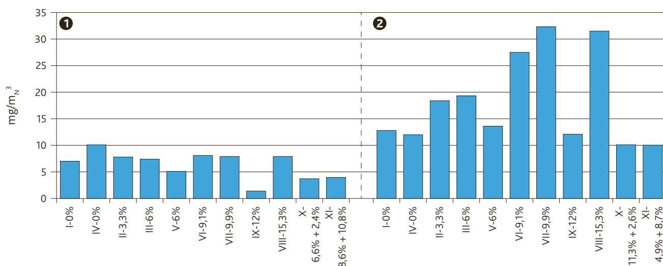
Слика 21. Емисије укупних прашкастих материја на мерним местима 1 и 2 у зависности од топлотног удела отпадних гума и отпадног уља у гориву
