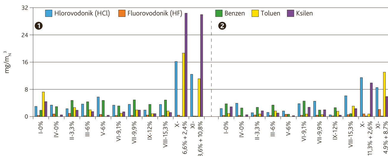
Слика 22. Емисије флуороводоника, бензена, хлороводоника, толуена и ксилена на мерним местима 1 и 2 у зависности од топлотног удела отпадних гума и отпадног уља у гориву
