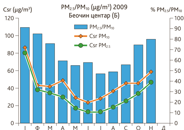
Слика 70. Средње месечне концентрације суспендованих честица PM_{2.5} и PM_{10} , Беочин-Центар, 2009.г., (оператер: СЕПА)
