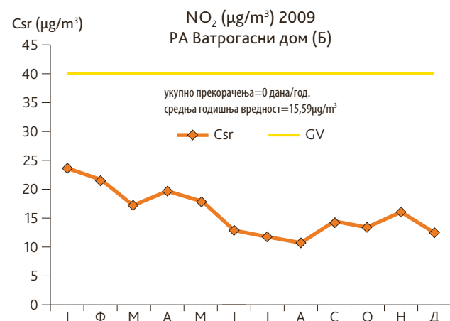
Слика 56. Годишњи тренд средњих месечних концентрација азот диоксида, Панчево-Ватрогасни дом, 2009.г., (оператер: ГПА)
