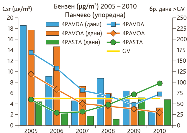
Слика 88. Упоредни годишњи тренд средњих месечних концентрација бензена и број дневних прекорачења граничних вредности, збирни преглед, Панчево, 2005-2010.
