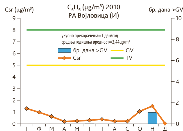
Слика 54. Годишњи тренд средњих месечних концентрација бензена и број дневних прекорачења граничних вредности, Панчево-Војловица, 2009.г., (оператер: ГПА)
