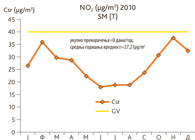
Слика 83. Годишњи тренд средњих месечних концентрација азот диоксида, Сремска Митровица, 2010.г., (оператер: СЕПА)
