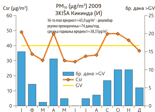
Слика 40. Годишњи тренд средњих месечних концентрација суспендованих честица PM_{10} и број дневних прекорачења граничних вредности, Кикинда, 2009.г. (оператер: ПСУГЗЖС)
