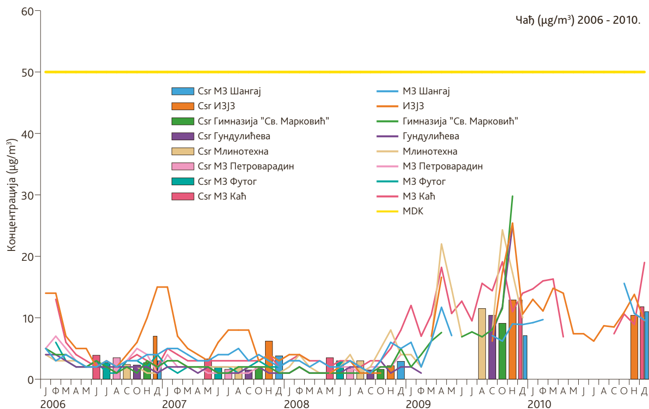
Слика 79. Средње месечне/годишње концентрације чађи, Нови Сад, 2006-2010 (извор: Институт за јавно здравље Војводине)
