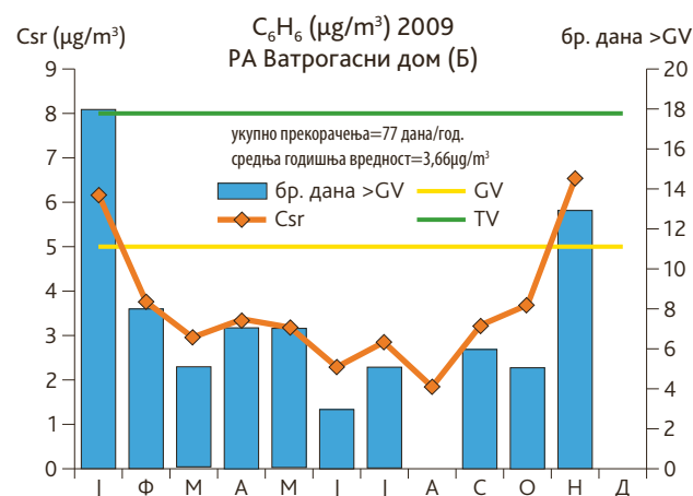
Слика 52. Годишњи тренд средњих месечних концентрација бензена и број дневних прекорачења граничних вредности, Панчево-Ватрогасни дом, 2009.г., (оператер: ГПА)
