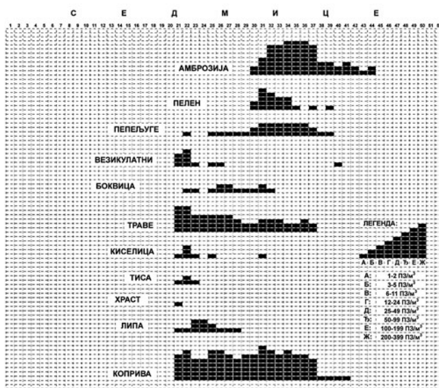
Слика 95. Календар аерополена у Сомбору у 2008.
