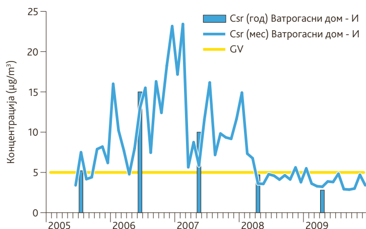
Слика 58. Средње месечне/годишње концентрације бензена, Панчево, 2005-2009
