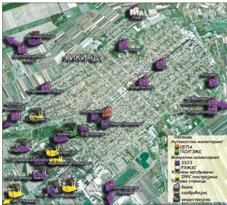
Слика 39. – Мрежа аутоматског и мануалног мониторинга у Севернобанатском округу
