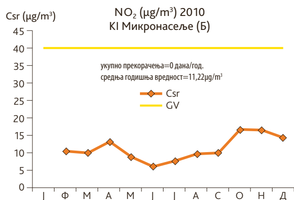
Слика 42. Годишњи тренд средњих месечних концентрација NO_2 , Кикинда, 2010.г. (оператер: СЕПА)
