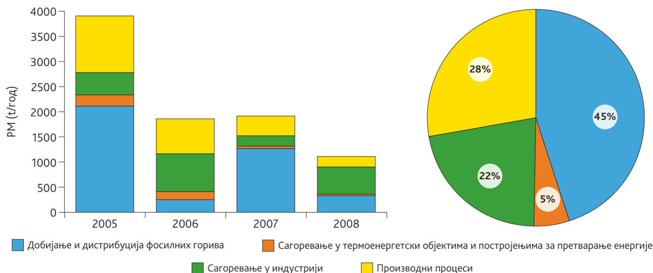
Слика 13. (лево) Емисије чврстих честица, из IPPC постројења по секторима, на територији АП Војводине у периоду од 2005. до 2008. године
