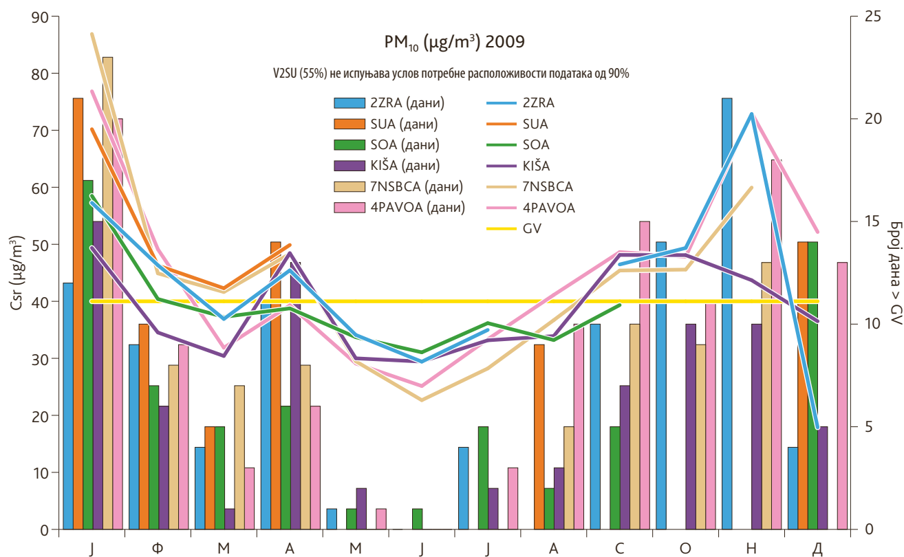
Слика 85. Упоредни годишњи тренд средњих месечних концентрација суспендованих честица PM 10 и број дневних прекорачења граничних вредности, збирни преглед, Војводина, 2009.
