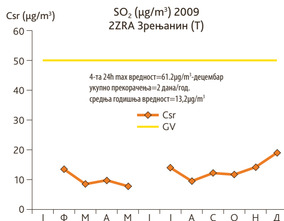
Слика 34. Годишњи тренд средњих месечних концентрација SO_2 , Зрењанин, 2009.г. (оператер: ПСУГЗЖС)
