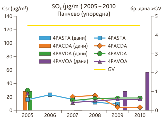
Слика 90. Упоредни годишњи тренд средњих месечних концентрација сумпор диоксида и број дневних прекорачења граничних вредности, збирни преглед, Панчево, 2005-2010.
