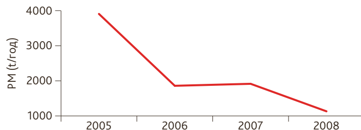
Слика 12. Тренд укупних емисија чврстих честица из IPPC постројења на територији АП Војводине у периоду од 2005. до 2008. године
