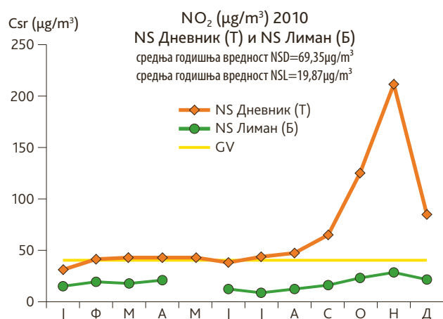
Слика 77. Упоредни годишњи тренд средњих месечних концентрација азот диоксида, Нови Сад-Дневник и Нови Сад-Лиман, 2010.г., (оператер: СЕПА)
