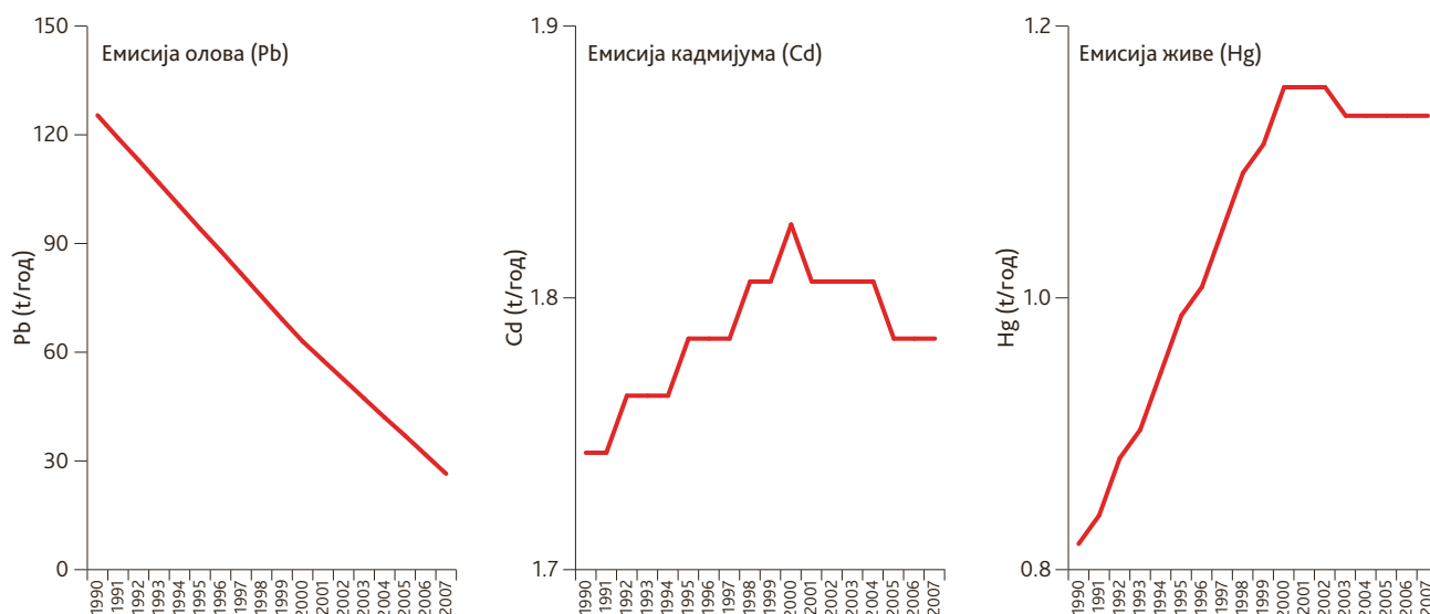
Слика 17. Тренд укупне процењене емисије олова (Pb), кадмијума (Cd) и живе (Hg) у АП Војводини у периоду од 1990. до 2007. године
