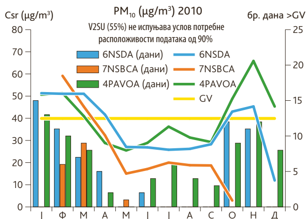
Слика 86. Упоредни годишњи тренд средњих месечних концентрација суспендованих честица PM_{10} и број дневних прекорачења граничних вредности, збирни преглед, Војводина, 2010.
