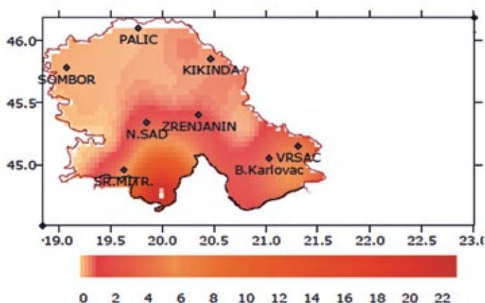
Слика 6. Билансиране емисије NO 2 , Gg, годишњи просек, од 1999 до 2003. године
