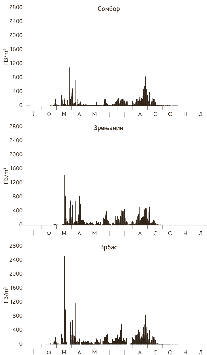
Слика 99. Варијација средњих дневних концентрација аерополену у Сомбору, Врбасу и Зрењанину у 2010. години
