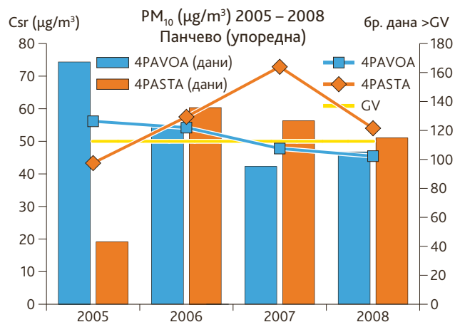
Слика 87. Упоредни годишњи тренд средњих месечних концентрација суспендованих честица PM_{10} и број дневних прекорачења граничних вредности, збирни преглед, Панчево, 2005-2008.
