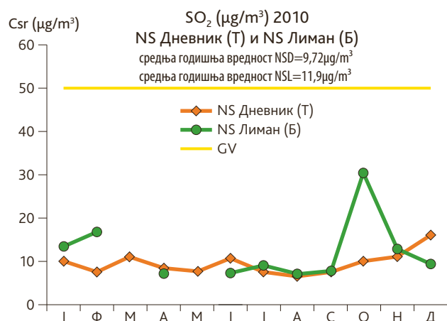
Слика 75. Упоредни годишњи тренд средњих месечних концентрација сумпор диоксида, Нови Сад-Дневник и Нови Сад-Лиман, 2010.г., (оператер: СЕПА)
