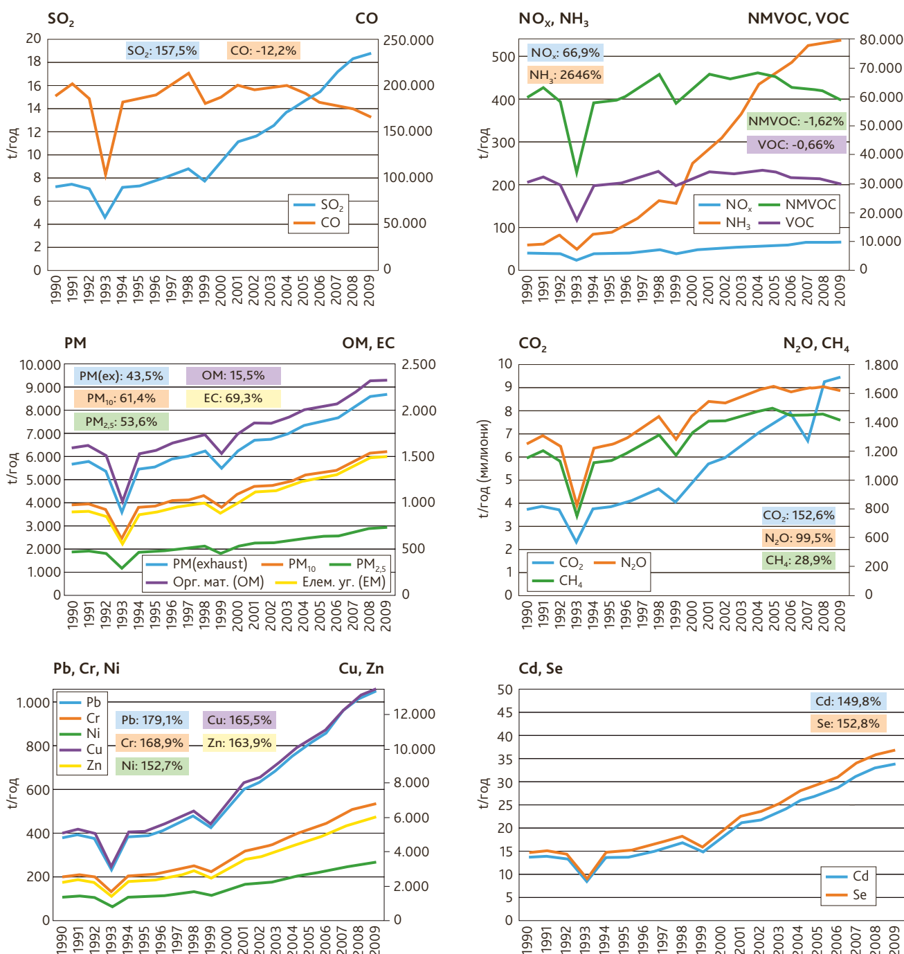
Слика 26. Тренд емисија из друмског саобраћаја (1990-2009)
