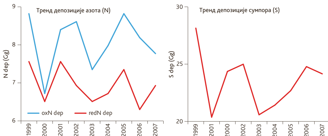
Слика 18. Тренд депозиције азота (N) и сумпора (S) на територији АП Војводине у периоду од 1999. до 2007. године
