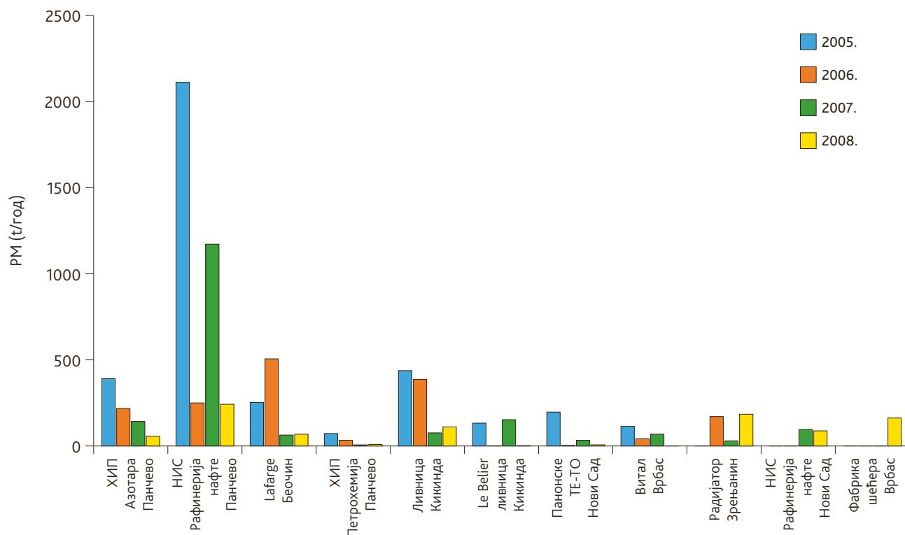
Слика 11. Емисије чврстих честица из IPPC постројења на територији АП Војводине у периоду од 2005. до 2008. године
