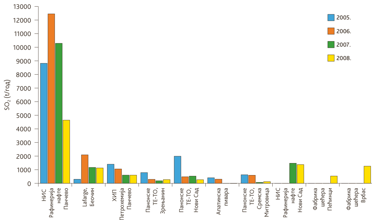
Слика 1. Емисије SO_2 из ИППС постројења на територији АП Војводине у периоду од 2005. до 2008. године
