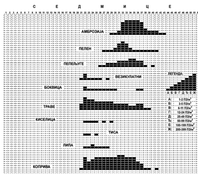
Слика 97. Календар аерополена у Зрењанину у 2008.
