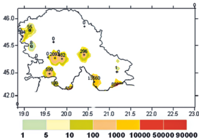
Слика 3. Емисије SO_2 током 2006. године у гриду 10 x 10 км
