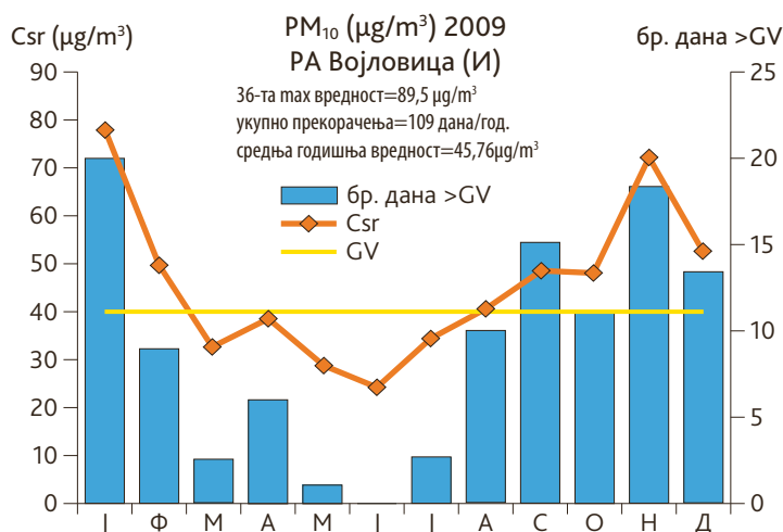
Слика 48. Годишњи тренд средњих месечних концентрација суспендованих честица PM 10 и број дневних прекорачења граничних вредности, Панчево-Војловица, 2009.г. (оператер: ГПА)
