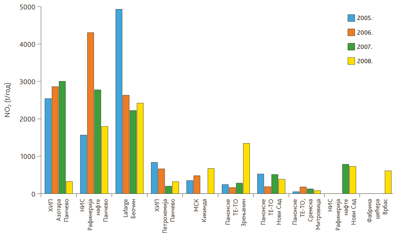
Слика 7. Емисије \text{NO}_2 из ИППС постројења на територији АП Војводине у периоду од 2005. до 2008. године
