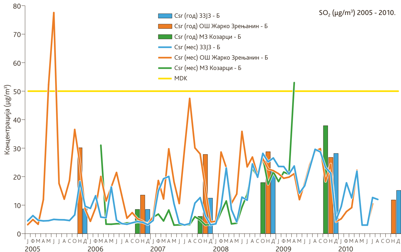
Слика 45. Средње месечне/годишње концентрације сумпор-диоксида, Кикинда 2005-2010 (Извор података: Завод за јавно здравље Кикинда)
