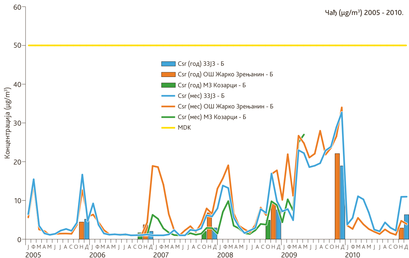
Слика 44. Средње месечне/годишње концентрације чађи, Кикинда 2005-2010 (Извор података: Завод за јавно здравље Кикинда)
