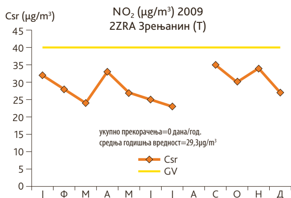
Слика 35. Годишњи тренд средњих месечних концентрација NO_2 , Зрењанин, 2009.г. (оператер: ПСУГЗЖС)
