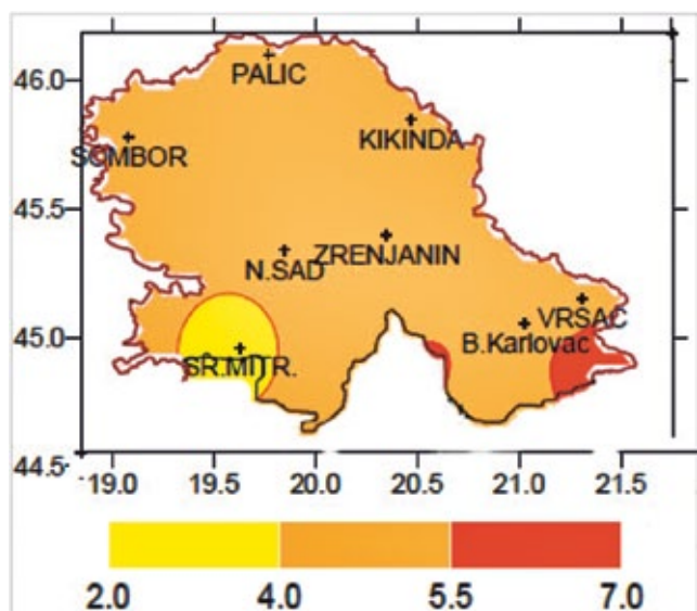
Слика 102. Територијална расподела тренда годишње температуре ваздуха °C/100год, у АП Војводина у периоду од 1991 до 2007. године
