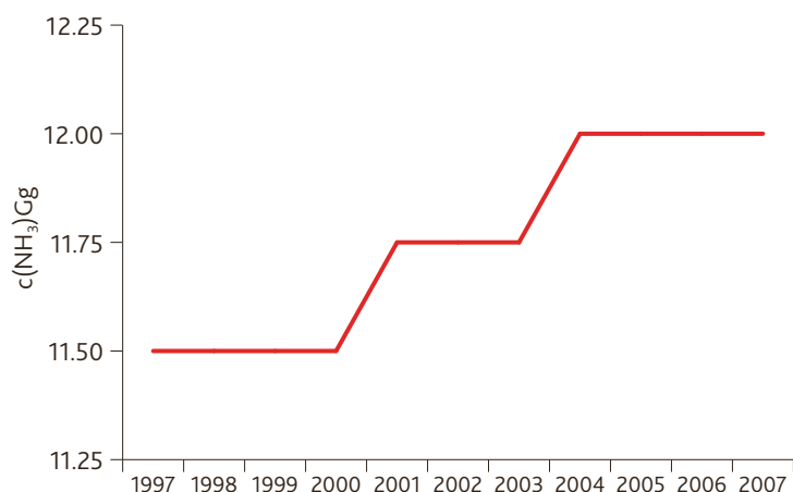
Слика 15. Процењене годишње емисије NH 3 (Gg) у АП Војводини у периоду од 1997. до 2007. године
