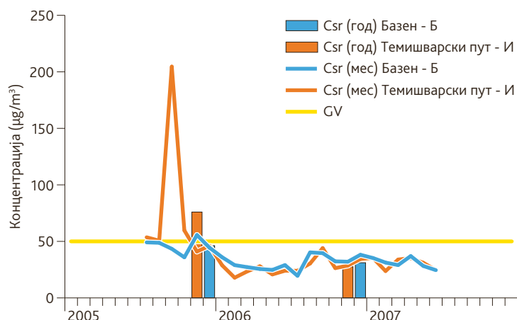
Слика 38. - Средње месечне/годишње концентрације сумпор-диоксида, Зрењанин 2005-2007. (Извор података: Завод за јавно здравље Зрењанин)
