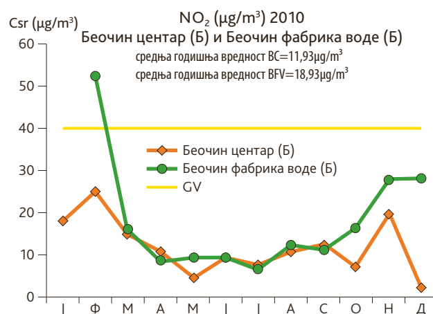
Слика 78. Упоредни годишњи тренд средњих месечних концентрација азот диоксида, Беочин, 2010.г., (оператер: СЕПА)
