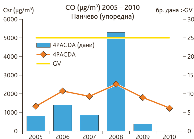
Слика 91. Упоредни годишњи тренд средњих месечних концентрација угљен монооксида и број дневних прекорачења граничних вредности, збирни преглед, Панчево, 2005-2010.
