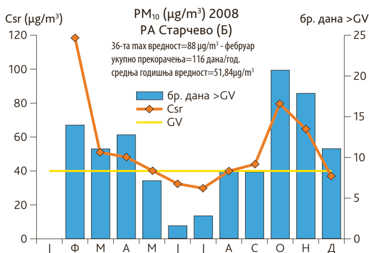
Слика 50. Годишњи тренд средњих месечних концентрација суспендованих честица PM 10 и број дневних прекорачења граничних вредности, Панчево-Старчево, 2008.г. (оператер: ГПА)
