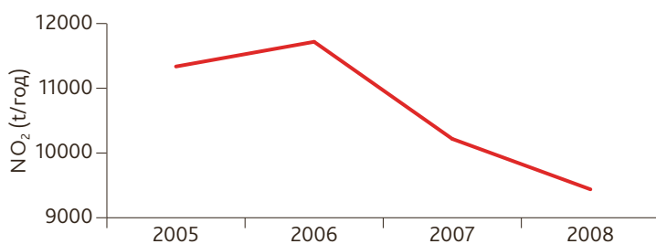
Слика 8. Тренд укупних емисија \text{NO}_2 из ИППС постројења на територији АП Војводине у периоду од 2005. до 2008. године
