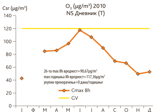
Слика 72. Годишњи тренд средњих месечних концентрација озона, Нови Сад-Дневник, 2010.г., (оператер: СЕПА)
