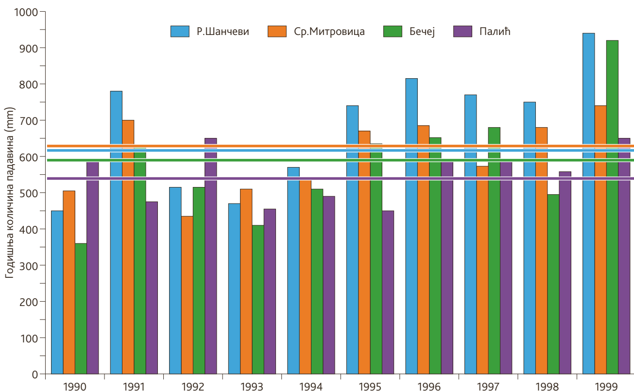
Слика 105. Годишња количина падавина у периоду од 1990. до 1999. године и средња годишња количина падавина на Римским Шанчевима, у Сремској Митровици и Бечеју и на Палићу (од 1948. до 1999. године)
