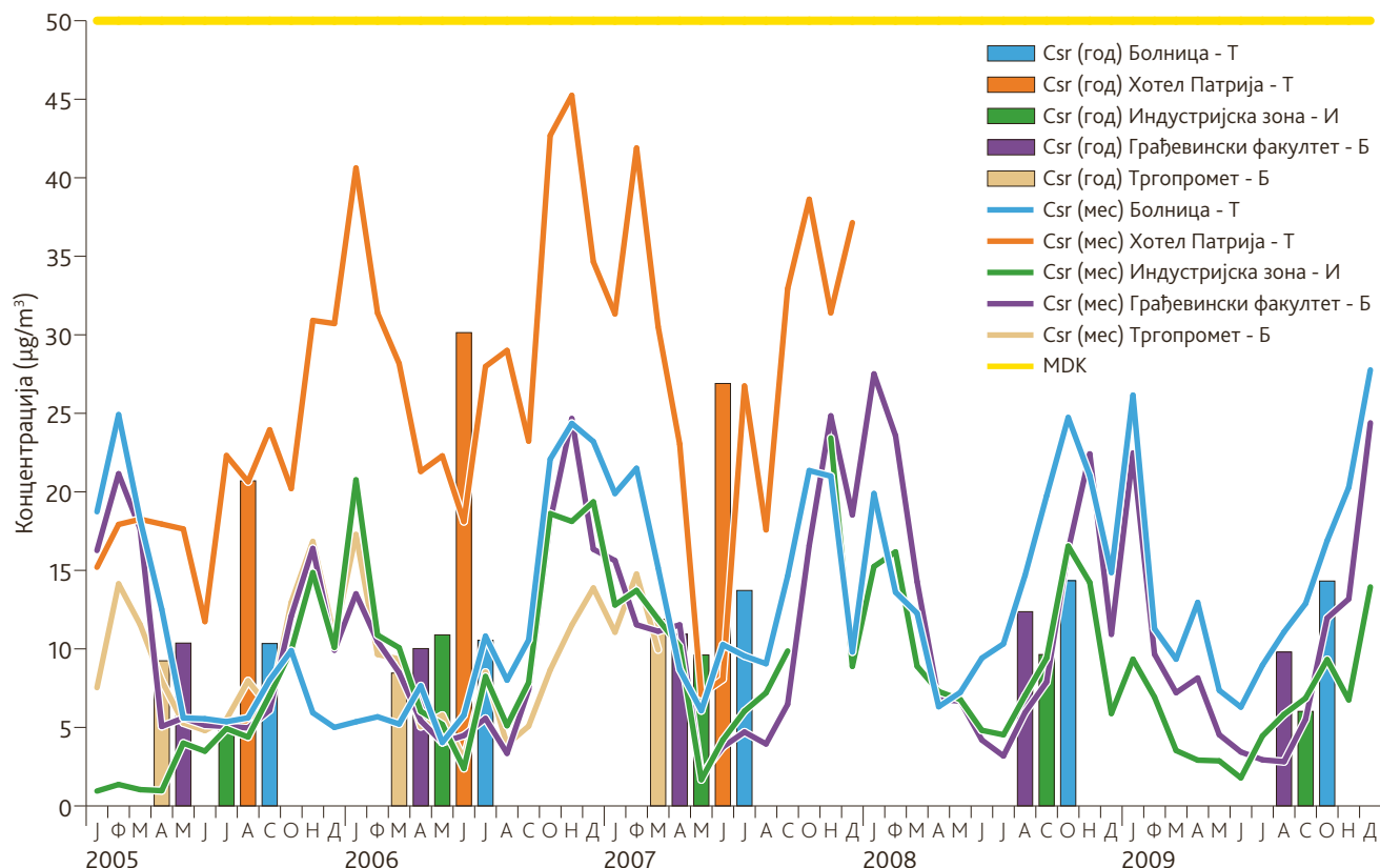
Слика 31. Средње месечне/годишње концентрације чађи, Суботица, 2005-2009. (Извор података: Завод за јавно здравље Суботице)
