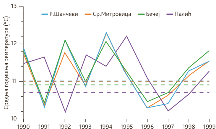
Слика 100. Промена средње годишње температуре ваздуха у периоду од 1990 до 1999. године и средња годишња температура ваздуха на Римским Шанчевима, у Сремској Митровици и Бечеју и на Палићу (1948-1999) (испрекидане линије)
