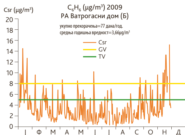
Слика 51. Средње дневне концентрације бензена, Панчево-Ватрогасни дом, 2009.г., (оператер: ГПА)
