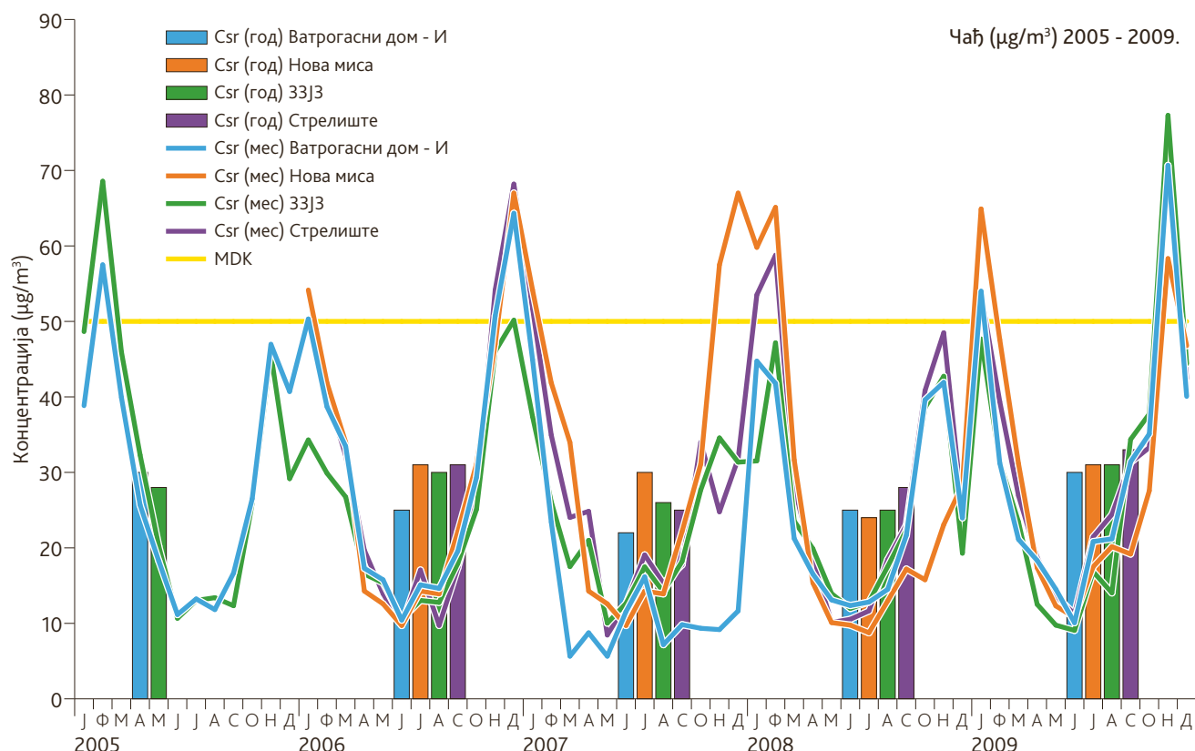
Слика 57. Средње месечне/годишње концентрације чађи, Панчево, 2005-2009
