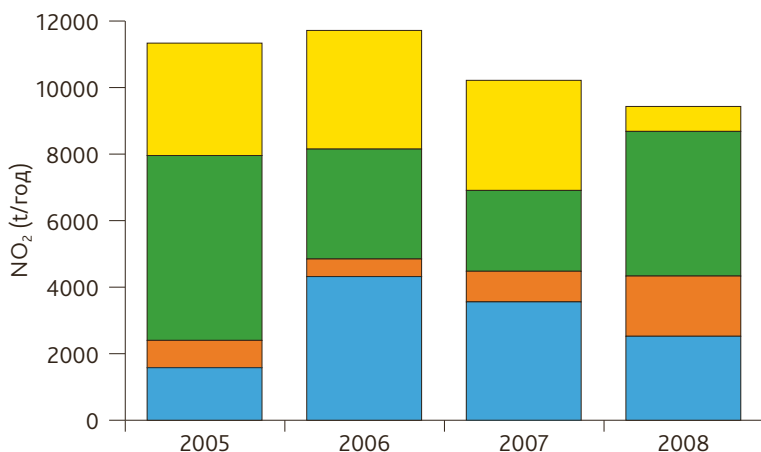
Слика 8. Тренд укупних емисија \text{NO}_2 из ИППС постројења на територији АП Војводине у периоду од 2005. до 2008. године
