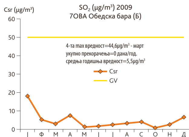
Слика 84. Годишњи тренд средњих месечних концентрација сумпор диоксида, Обедска бара, 2010.г., (оператер: ПСУГЗЖС)
