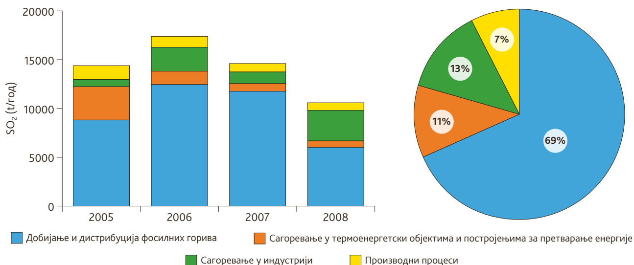
Слика 4. (лево) Емисије SO 2 из IPPC постројења по секторима, на територији АП Војводине, у периоду од 2005. до 2008. године Слика 5. (десно) Укупни удели емисија SO 2 из IPPC постројења, по секторима, на територији АП Војводине, у периоду од 2005. до 2008. године
