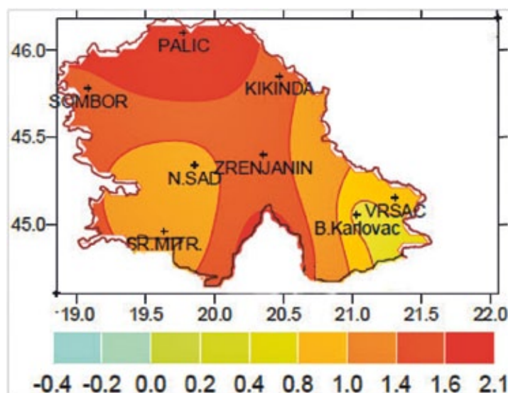
Слика 101. Територијална расподела тренда годишње температуре ваздуха °C/100год, у АП Војводина у периоду од 1951 до 2007. године
