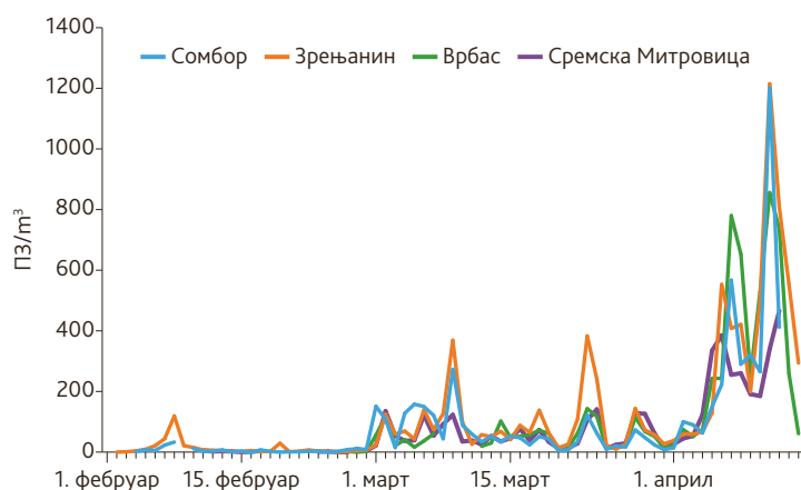
Слика 98. Графички приказ варијација дневних концентрација аерополену у Сомбору, Зрењанину, Врбасу и Сремској Митровици (1. фебруар-15. април 2009. г.)
