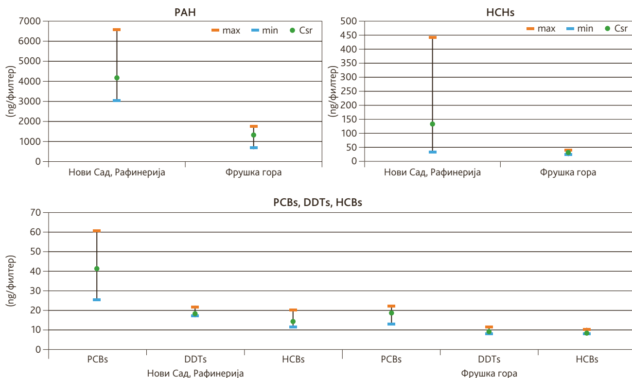
Слика 92. Концентрације PCBs, HCHs, DDTs, HCBs и PAHs одређених у пасивно узоркованом узорку ваздуха на локацијама Рафинерија нафте Нови Сад и Фрушка гора
