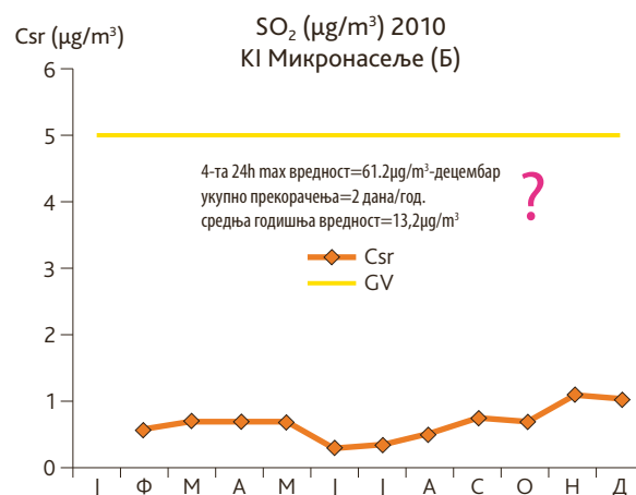
Слика 41. Годишњи тренд средњих месечних концентрација SO_2 , Кикинда, 2010.г. (оператер: СЕПА)
