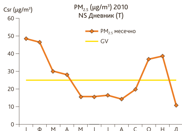
Слика 66. Годишњи тренд средњих месечних концентрација суспендованих честица PM_{2.5} , Нови Сад-Дневник, 2010.г., (оператер: СЕПА)
