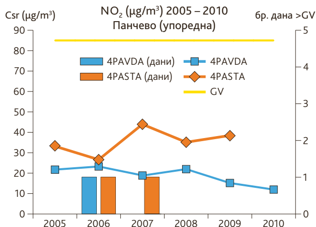
Слика 89. Упоредни годишњи тренд средњих месечних концентрација азот диоксида и број дневних прекорачења граничних вредности, збирни преглед, Панчево, 2005-2010.
