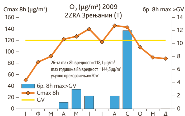
Слика 36. Годишњи тренд средњих месечних концентрација O_3 и број прекорачења граничних вредности 8-х тах, Зрењанин, 2009.г. (оператер: ПСУГЗЖС)
