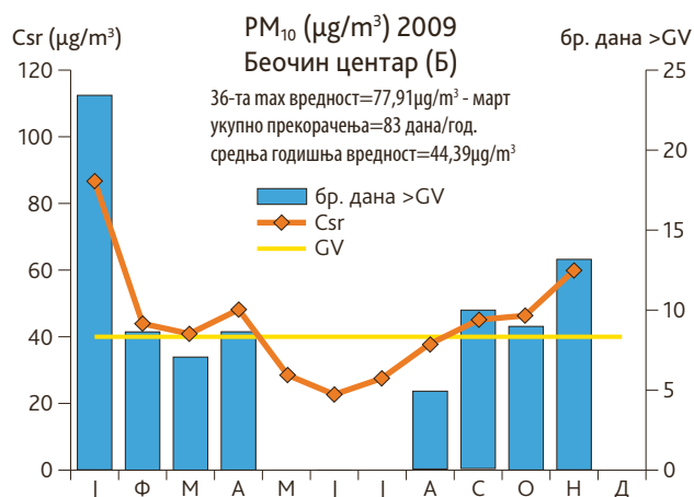
Слика 68. Годишњи тренд средњих месечних концентрација суспендованих честица PM_{10} и број дневних прекорачења граничних вредности, Беочин-Центар, 2009.г., (оператер: СЕПА)
