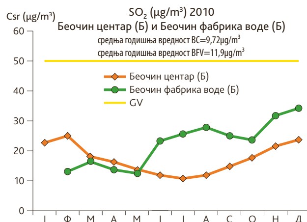
Слика 76. Упоредни годишњи тренд средњих месечних концентрација сумпор диоксида, Беочин, 2010.г., (оператер: СЕПА)
