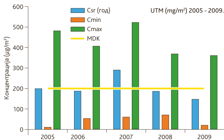
Слика 63. Средње годишње концентрације укупних таложних материја, Сомбор, 2005-2009.
