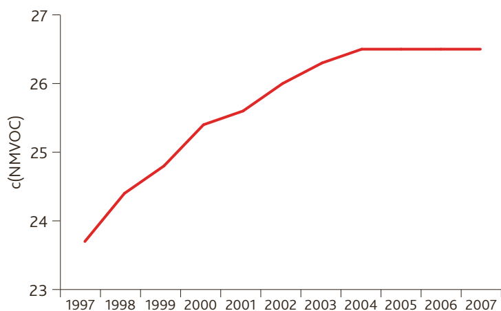
Слика 16. Процењене годишње емисије неметанских испарљивих органских једињења (NMVOCs) (Gg) у АП Војводини у периоду од 1997. до 2007. године
