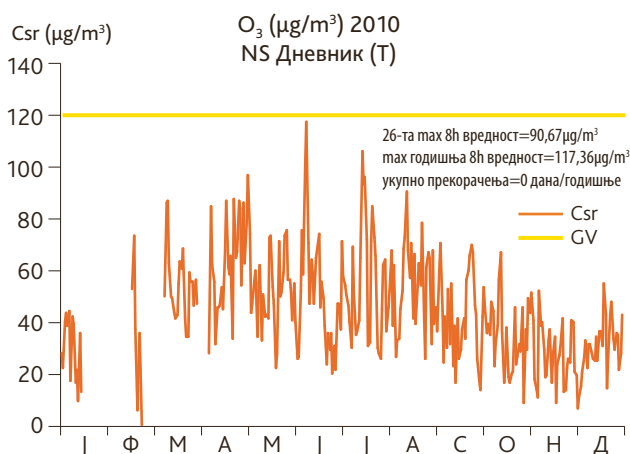
Слика 71. Средње дневне концентрације озона, Нови Сад-Дневник, 2009.г., (оператер: СЕПА)
