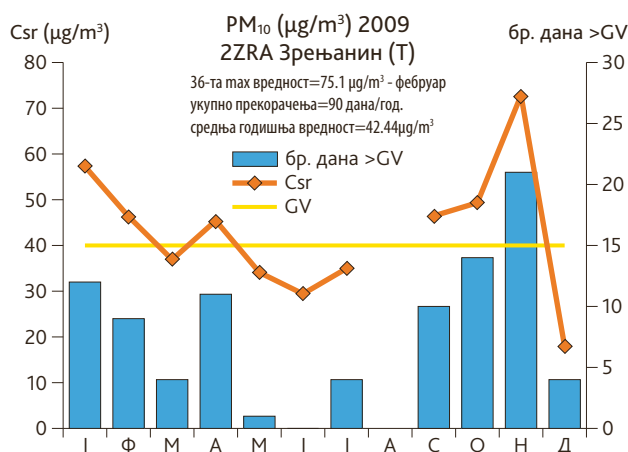
Слика 33. Годишњи тренд средњих месечних концентрација суспендованих честица PM_{10} и број дневних прекорачења граничних вредности, Зрењанин, 2009.г. (оператер: ПСУГЗЖС)
