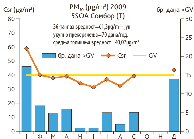
Слика 61. Годишњи тренд средњих месечних концентрација суспендованих честица PM_{10} и број дневних прекорачења граничних вредности, Сомбор, 2009.г. (оператер: ПСУГЗЖС)
