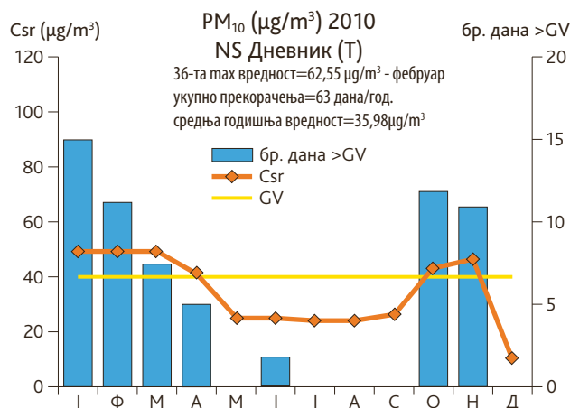
Слика 65. Годишњи тренд средњих месечних концентрација суспендованих честица PM_{10} и број дневних прекорачења граничних вредности, Нови Сад-Дневник, 2010.г., (оператер: СЕПА)
