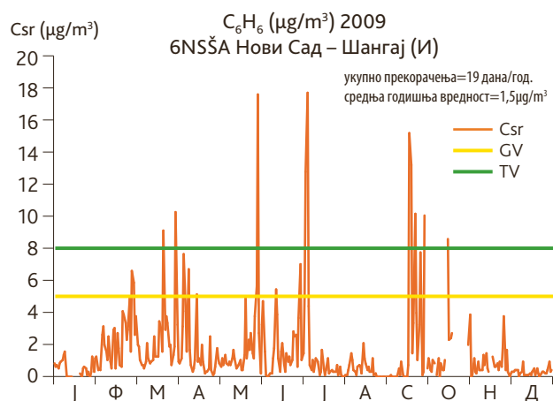
Слика 73. Средње дневне концентрације бензена, Нови Сад-Шангај, 2009.г., (оператер: ПСУГЗЖС)
