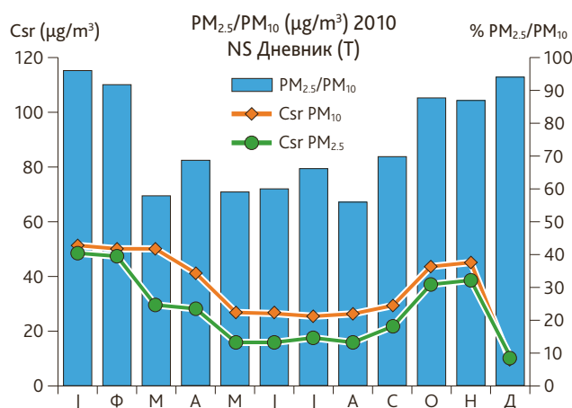
Слика 67. Средње месечне концентрације суспендованих честица PM_{2.5} и PM_{10} , Нови Сад-Дневник, 2010.г., (оператер: СЕПА)
