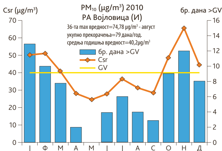
Слика 49. Годишњи тренд средњих месечних концентрација суспендованих честица PM 10 и број дневних прекорачења граничних вредности, Панчево-Војловица, 2010.г. (оператер: ГПА)
