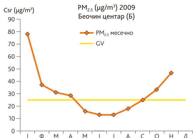
Слика 69. Годишњи тренд средњих месечних концентрација суспендованих честица PM_{2.5} , Беочин-Центар, 2009.г., (оператер: СЕПА)
