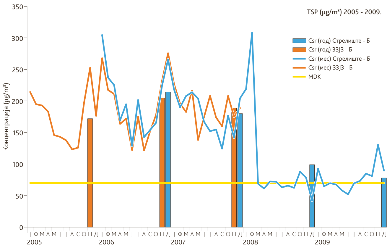
Слика 59. Средње месечне/годишње концентрације укупних суспендованих честица, Панчево, 2005-2009
