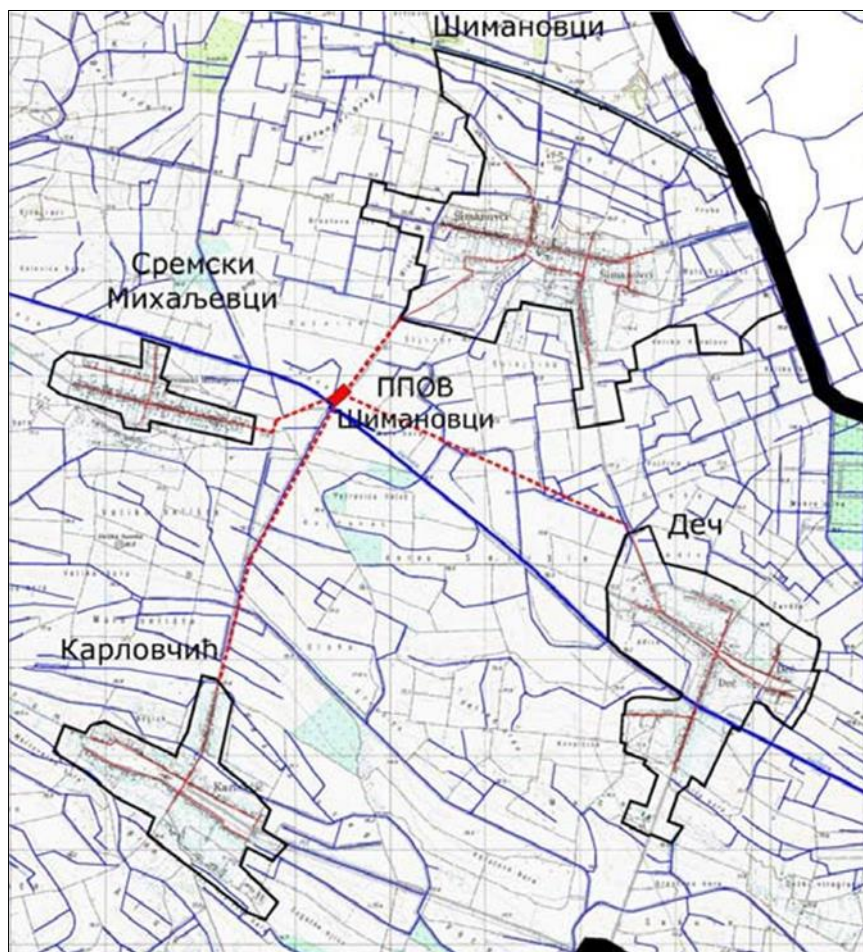
Слика 22. Међумесни систем ППОВ Шимановци - ситуација
