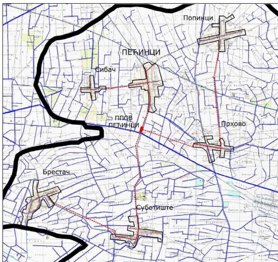
Слика 21. Међумесни систем ПОВ Пејинци - ситуација
