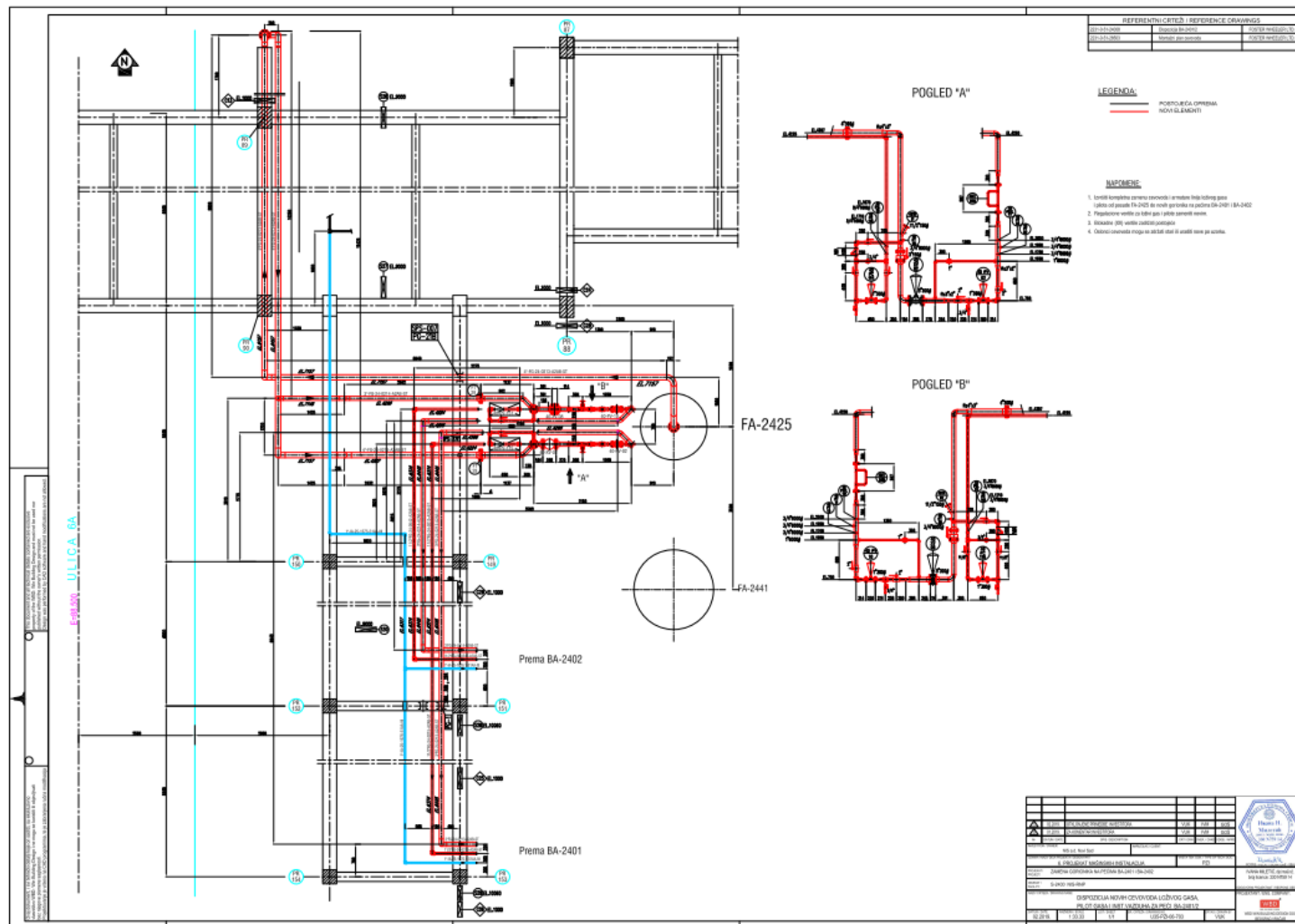
Slika 3.1.1. Dispozicija novih cevovoda loživog gasa, pilot gasa i instrumentalnog vazduha za peći BA-2401/2
