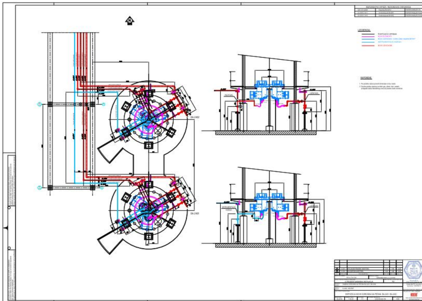
Slika 3.1.2. Dispozicija novih gorionika na pećima BA-2401 i BA-2402
