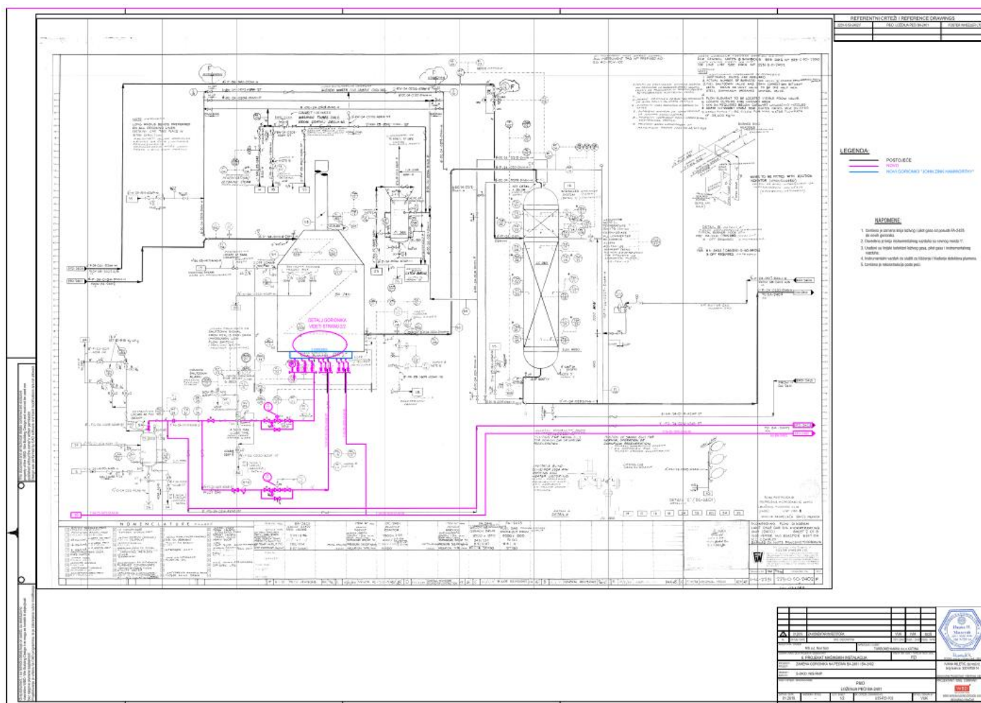
Slika 3.2.1. P&ID Loženja peći BA-2401 (str. 1/2)
