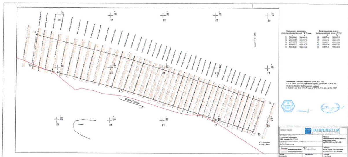
Слика 1: Катастарско-топографски план за снимљену локацију на реци Дунав км 1262+000 до км 1263+000, у К.О. Ветерник, Лединци и обухват багерована.
