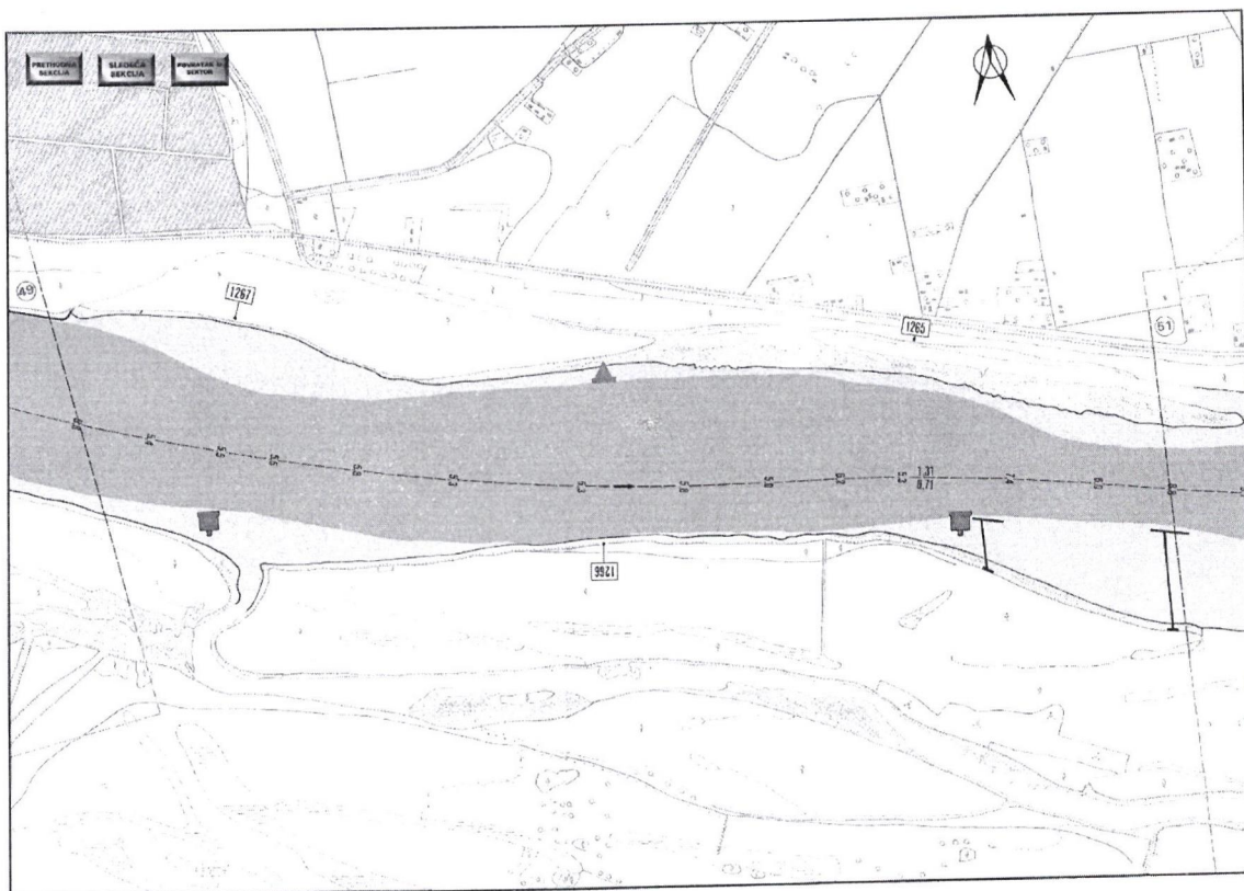
Slika 3. Situacija lokacije reke Dunav od km 1266+700 do km 1267+200
