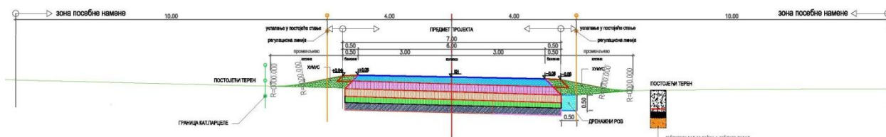
1 профил - каблови положени поред главног приступног пута
