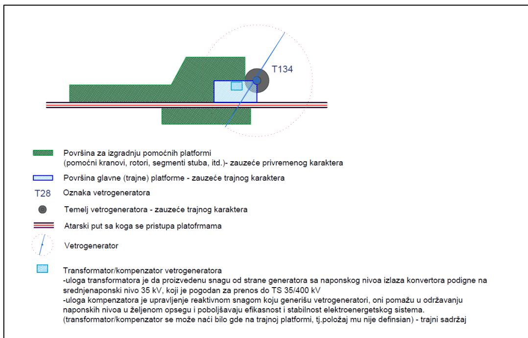
Слика 9. Шематски приказ типске организације ветрогенератора са садржајима – трајна платформа у односу на приступни пут
