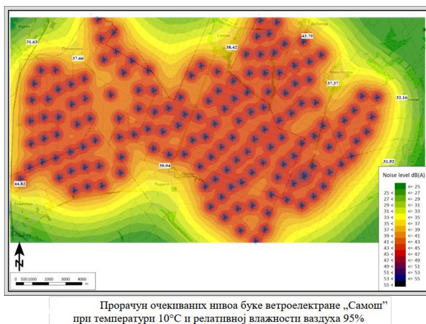
Слика 4: Расподела нивоа буке у околини будуће ветроелектране „Самош“
