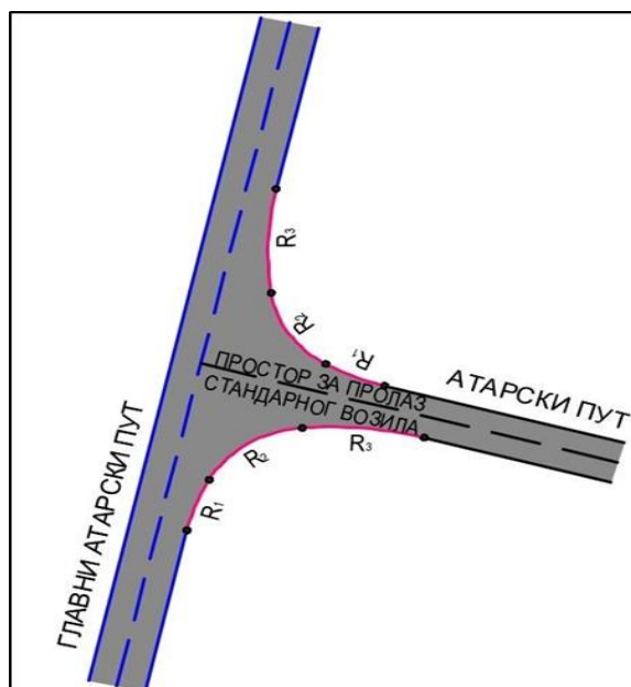
Слика 6: Детаљ раскрснице за пролазак стандардних возила
