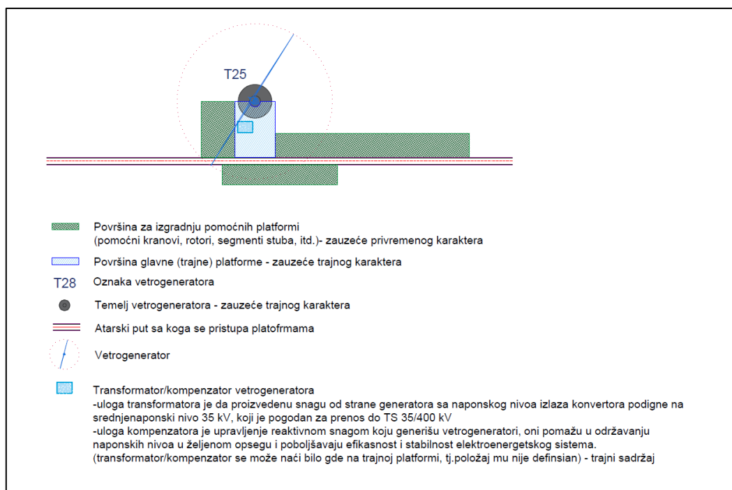
Слика 10. Шематски приказ типске организације ветрогенератора са садржајима – трајна платформа управна у односу на приступни пут
