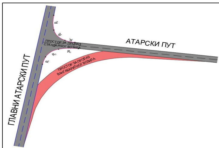
Слика 7: Детаљ раскрснице за пролазак вангабаритних возила
