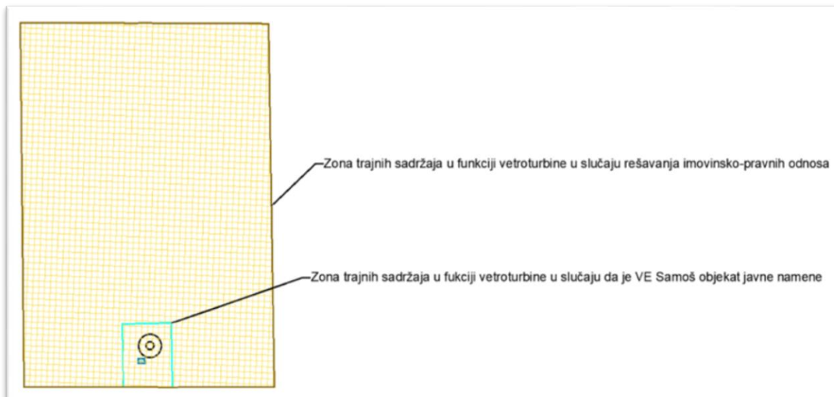
Слика 8. Зоне трајних садржаја у функцији ветрогенератора
