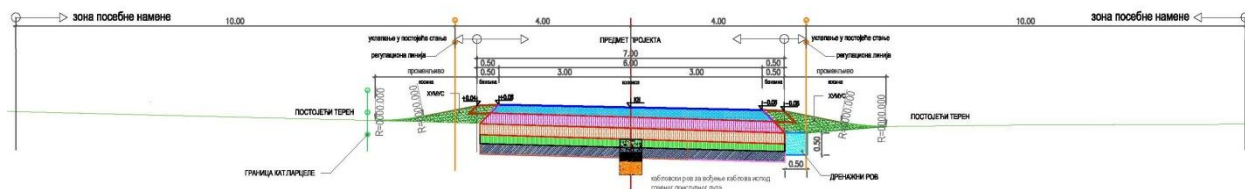
2 профил - каблови положени испод главног приступног пута
