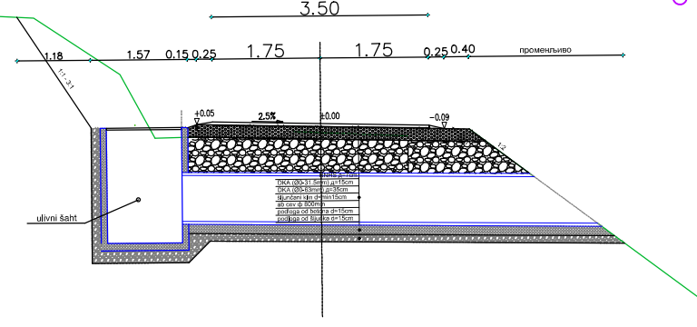
НОРМАЛНИ ПОПРЕЧНИ ПРОФИЛ 4 - 4
