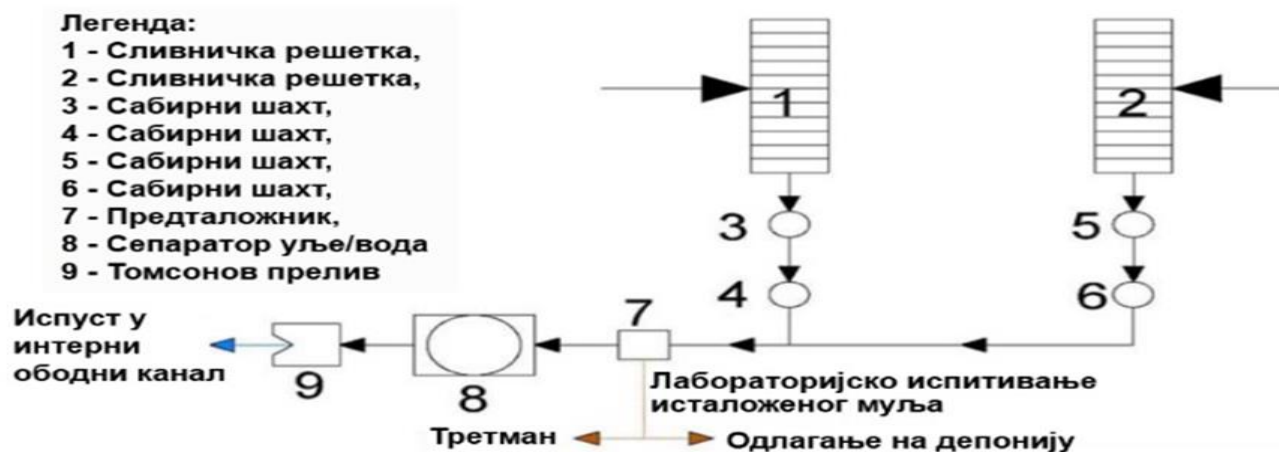
Слика 10. Технолошка шема токова атмосферске зауљене воде
