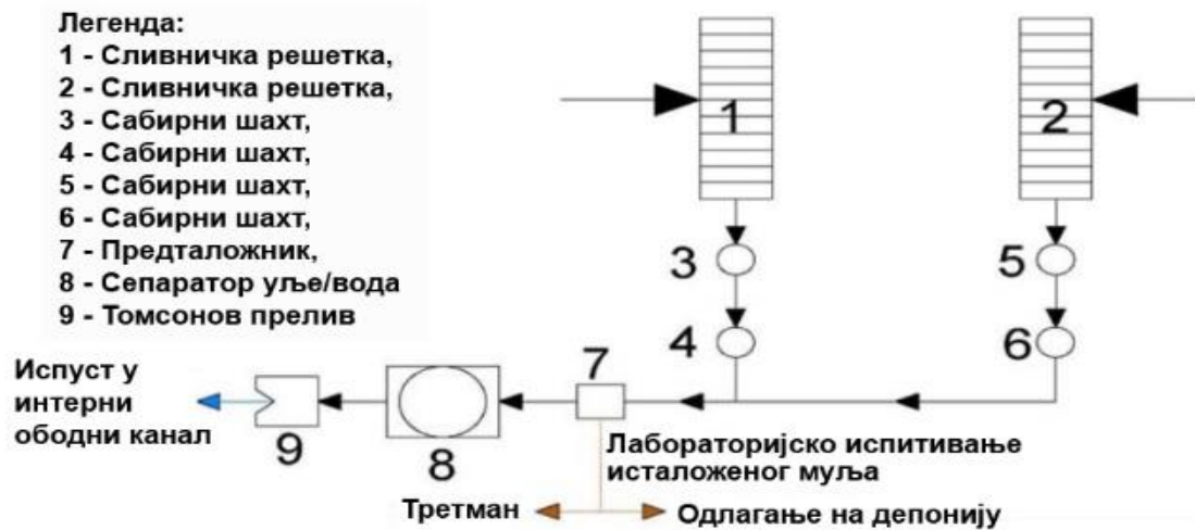
Слика 4. Технолошка шема токова атмосферске зауљене воде
